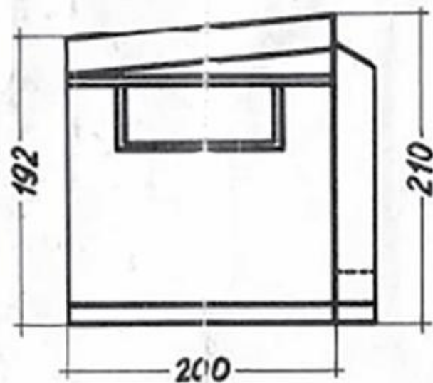
Seitenansicht side-view
