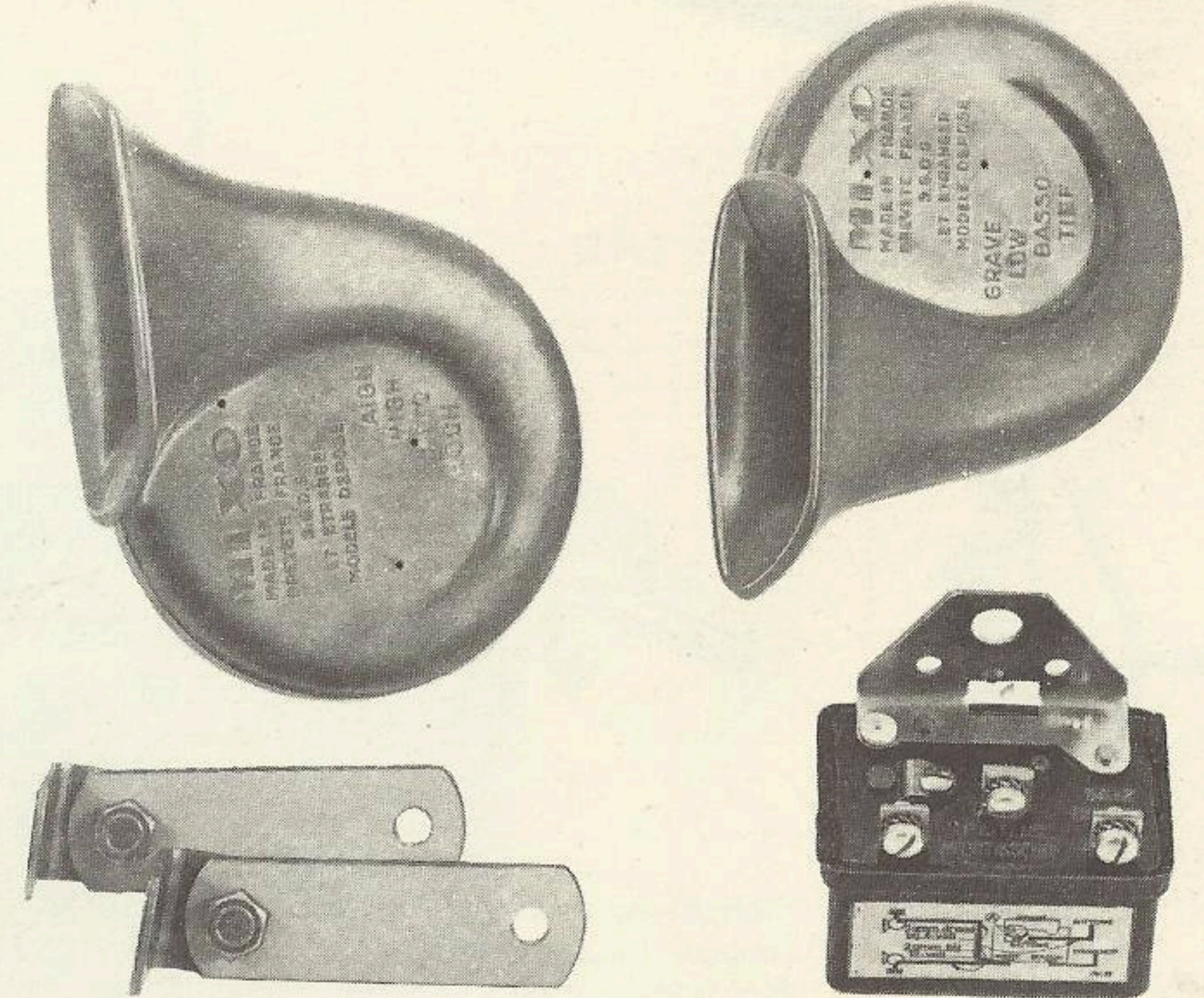
Dubbeltonige elektrische claxons van de merken: „Bosch”, „Hella” en „Mixo” in 6 of 12 Volt.
